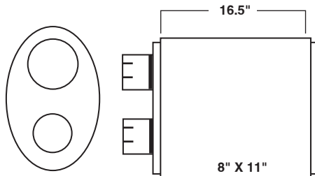
MODEL: CAT D4
